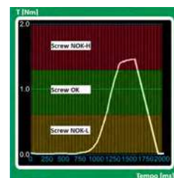
Visualizzazione degli esiti di avvitatura: tavola di riferimento Viewing of tightening results: reference table
